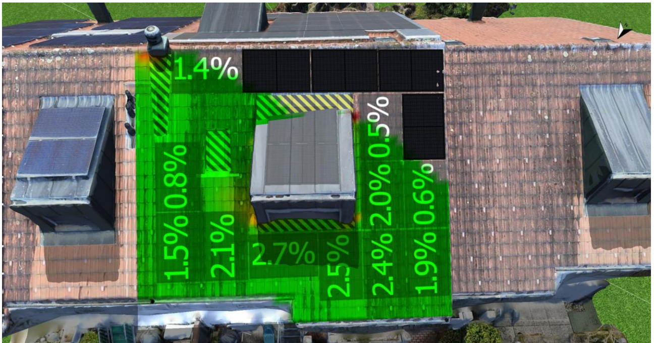
Verschattungssimulation
