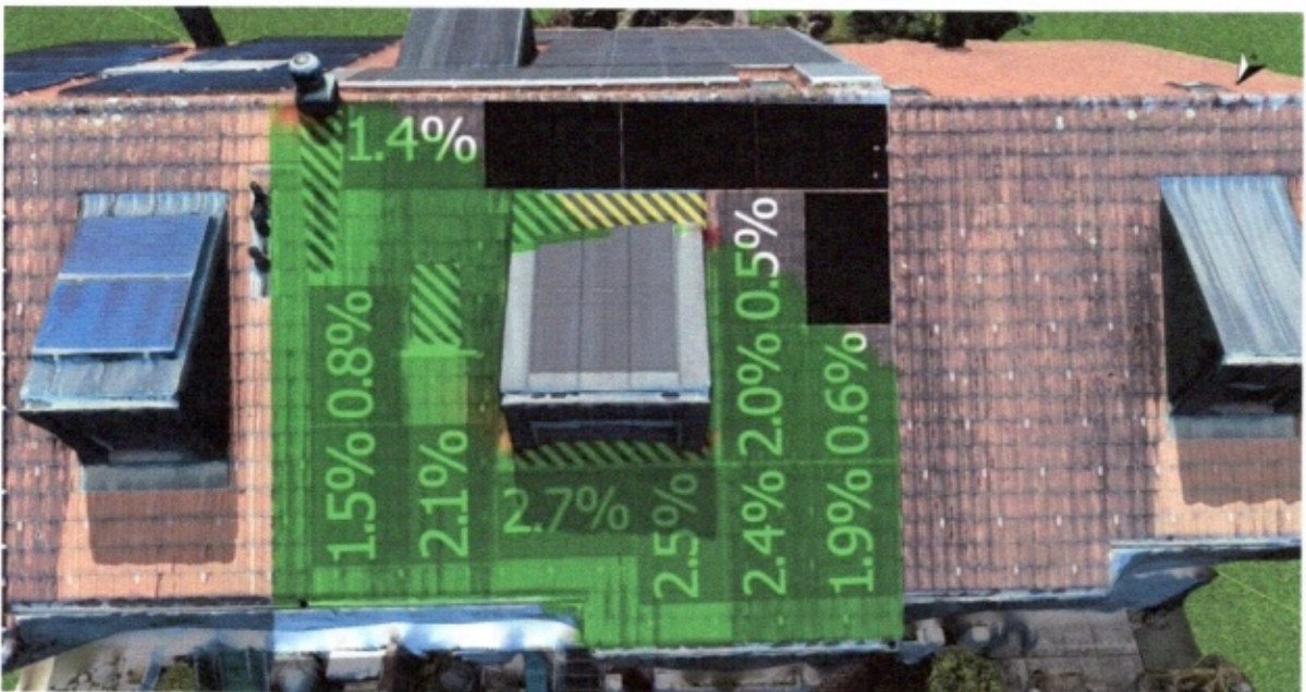
Verschattungssimulation
