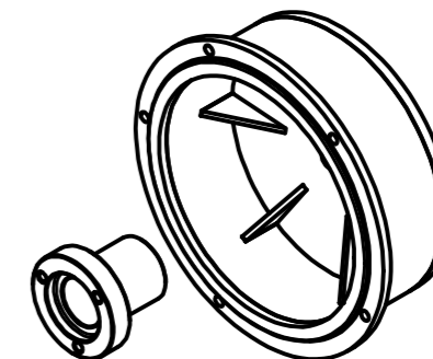
1080960211 UTIL CIGÜEÑAL TR280i
