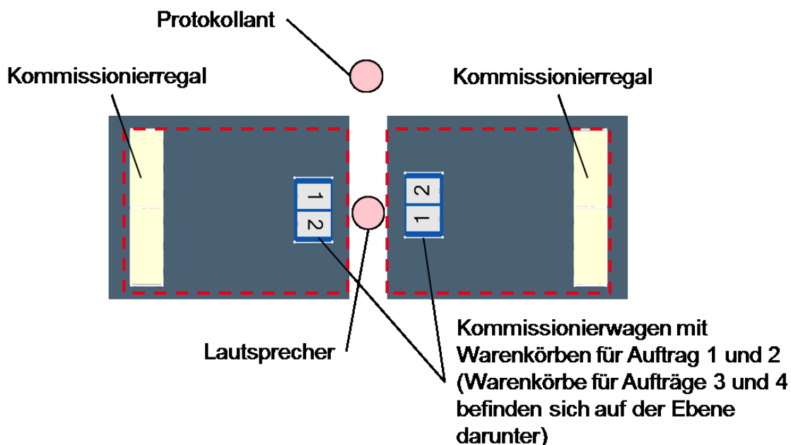
Abbildung 17: Draufsicht der erweiterten Kommissionierumgebung in der realen Umgebung (eigene Darstellung)
