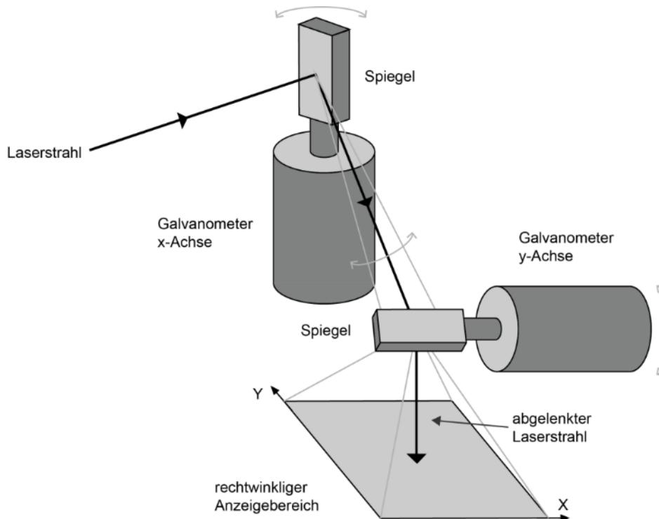
Abbildung 7-9: Funktionsweise der Strahlableitung eines Laserprojektors
