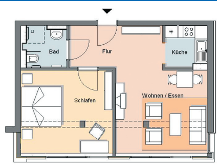
Beispielgrundriss Zweizimmerwohnung
