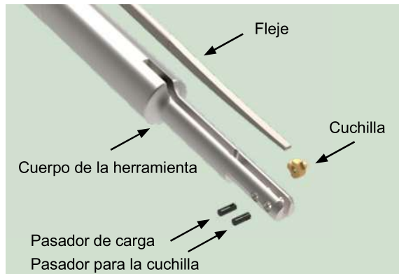
Imagen 4: para el cambio de cuchilla retire solo el primer pasador que sujeta la cuchilla.
