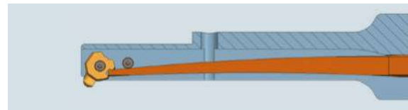
Imagen 3: El fleje precargado y el mango rebajado permite el rebabado de agujeros con alto grado de irregularidad.
