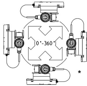
Abb. 4: Einbaupositionen
