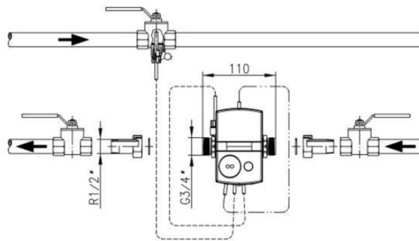
Abb. 5: Installationsbeispiel
