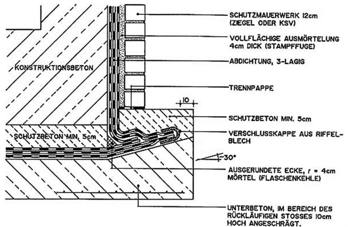
Bild 3 Rückläufiger Stoß
