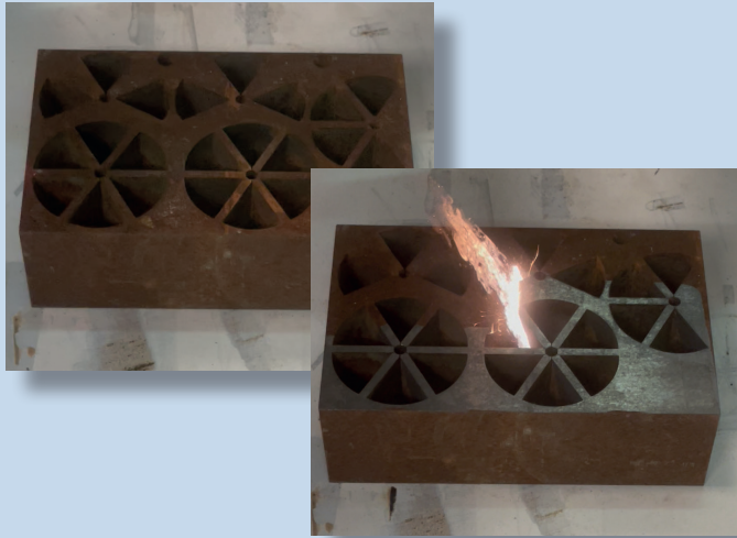
Avant / après sur pièce en acier PT 110Kg
