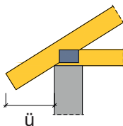
schräger Überstand
