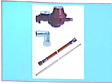
Nr. 0207010 Herdanschluß-Set 1,5kg 50mbar Schl. 400 mm + Zubeh.
