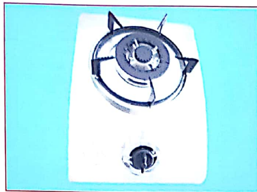
Nr. HW2113 Wokbrenner 3,7kw Edel. m. Zünd. + autom. Zünd. nur Propan
