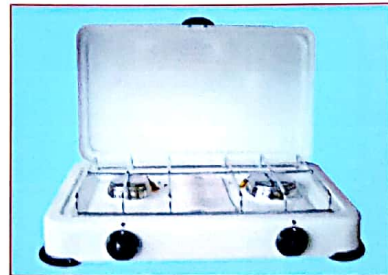
Nr. K2352 Kocher 2 Fl. m. Zünds. Chromrost weiß nur Propan H10 B48 T30
