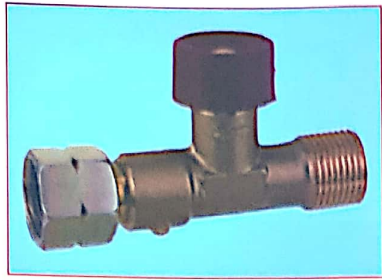
Nr. 0282502 Schlauchbr. 1,5bar 3kg 3/8L
