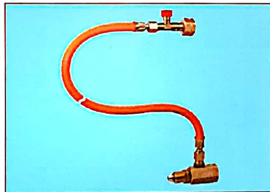
Nr. 02499 Notversorgungs-Garnitur PN25 kompl. SBSKomb. Ax2000mm
