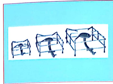
Nr. HK141173A / Nr. HK14117B / Nr. HK14117C Hockerkocher o. Zünds. 2,5kw, 6kw, 9,2kw nur Propan H12 B21 T27, H30 B30 T40, H40 B20 T50
