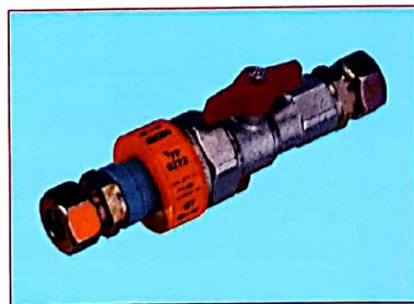
Nr. 02713 Kugelhahn m. Isostück beids. 18x18 Schn. vor Hausenf.
