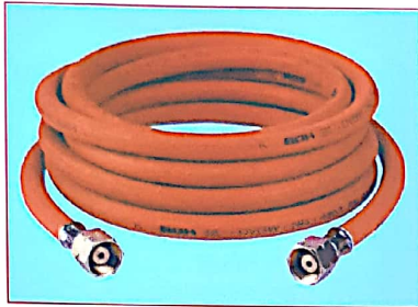
Nr. 04502 / Nr. 04503 / Nr. 04504 Nr. 04506 / Nr. 04511 Schl. 6,3x3,5 3/8 x 3/8Lx1500mm Schl. 6,3x3,5 3/8 x 3/8Lx2000mm Schl. 6,3x3,5 3/8 x 3/8Lx3000mm Schl. 6,3x3,5 3/8 x 3/8Lx5000mm Schl. 6,3x3,5 3/8 x 3/8Lx10000mm
