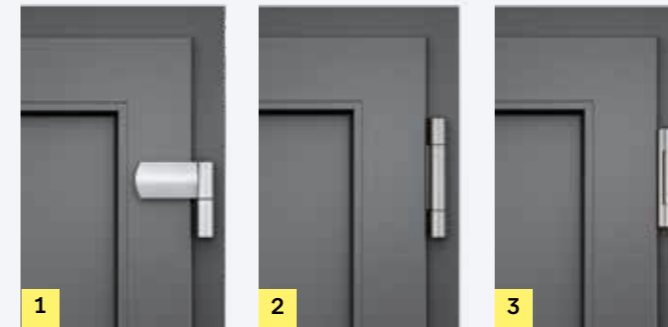
1 | Aufschraubband. (WERU AVIDA) 2 | Rollenband. (WERU AVIDA) 3 | Aufschraubrollenband (WERU TERSA)
