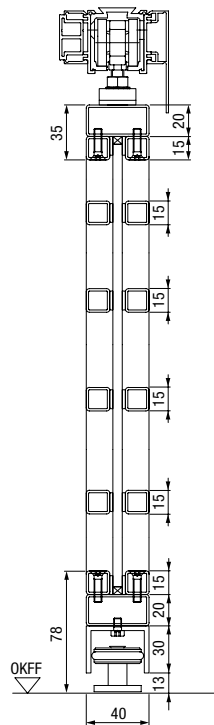
Vertikalschnitt 1-flügelige Stahl-Lofttür
