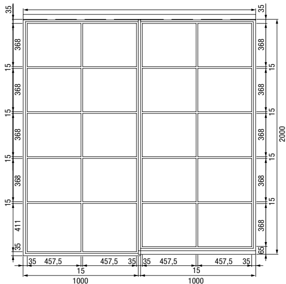
1-flügelige Stahl-Lofttür mit Seitenteil
