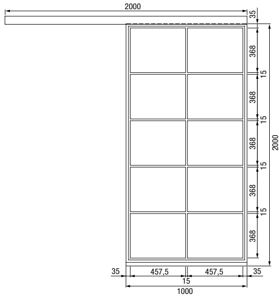
1-flügelige Stahl-Lofttür
