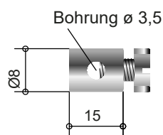
Schraubnippel mit Sechskantschraube und Schlitz
