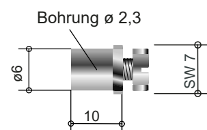
Schraubnippel mit Schlüsselansatz und Sechskantschraube
