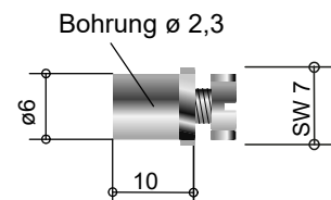
Schraubnippel mit Schlüsselansatz und Sechskantschraube
