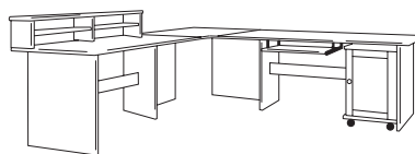
BEISPIEL 4 Breite: 228,5/263,5 x Höhe: 74 x Tiefe: 78 cm
